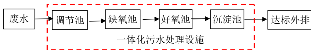
图 5-2 生活污水处理设施工艺流程图
