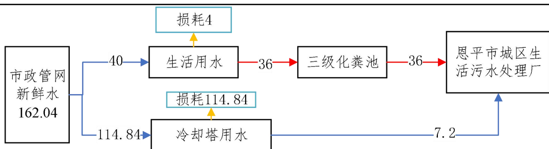
图 1 本改扩建项目水平衡图 (m 3 /a)
