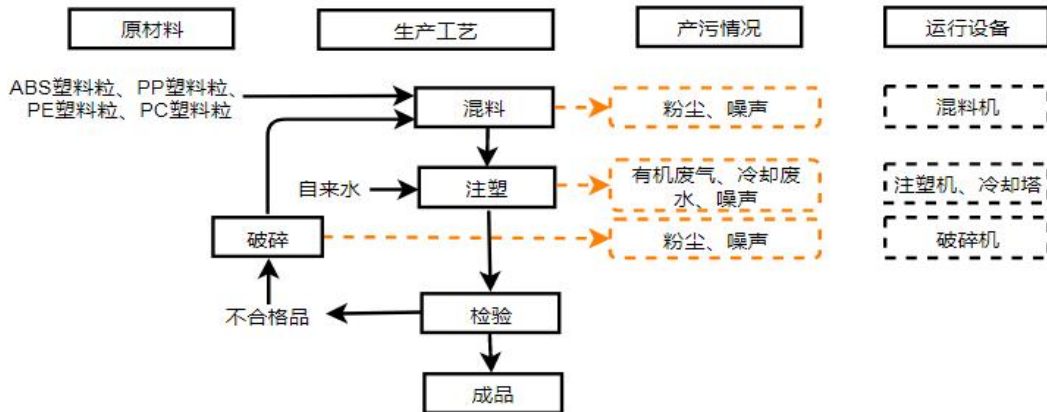
图 2 本改扩建项目产品生产工艺流程及产污过程图
