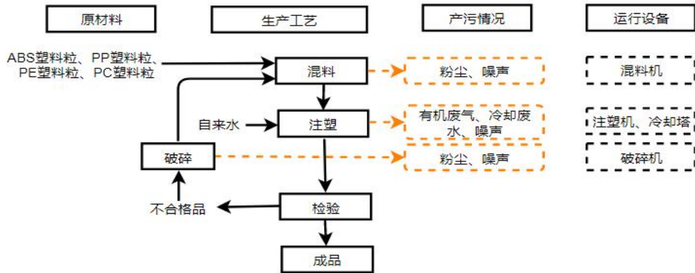
图3 项目产品（麦克风塑料配件）生产工艺流程及产污环节图
