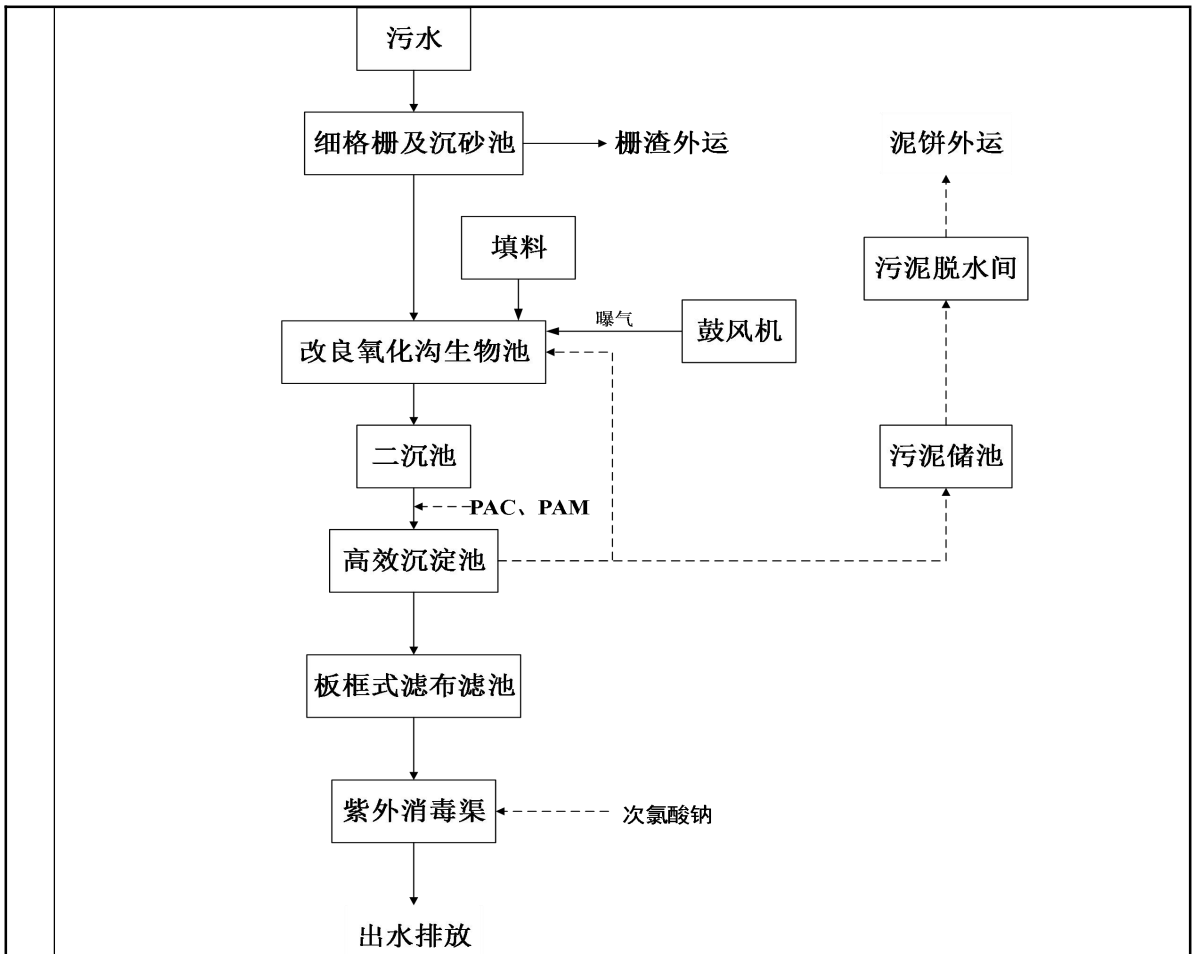
图 6 恩平市城区生活污水处理厂工艺流程图
