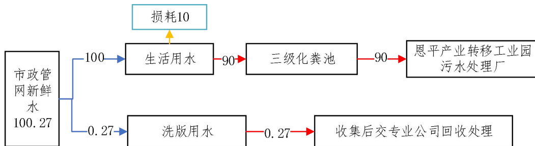
图 1 项目后的项目水平衡图（单位 \text{m}^3/\text{a} ）
