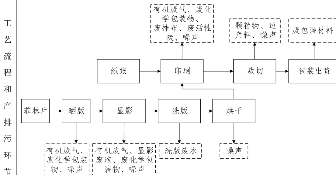
图 2 项目纸制品印刷生产工艺流程及产污过程图
