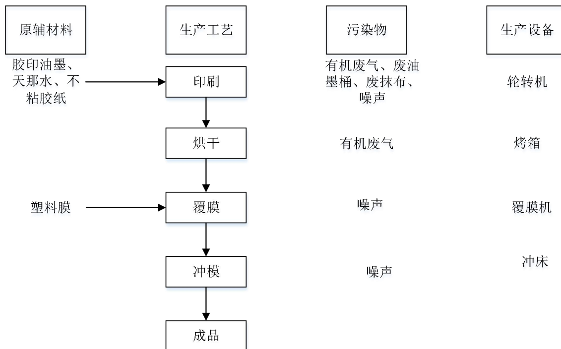
图2-4丝印不粘胶纸生产工艺及产污环节示意图
