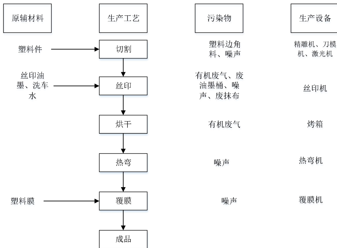
图2-3塑料丝印制品生产工艺及产污环节示意图
