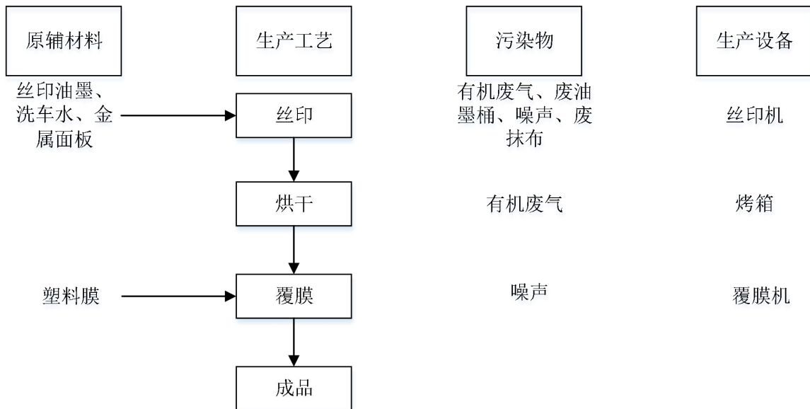
图 2-2 金属丝印制品生产工艺及产污环节示意图
