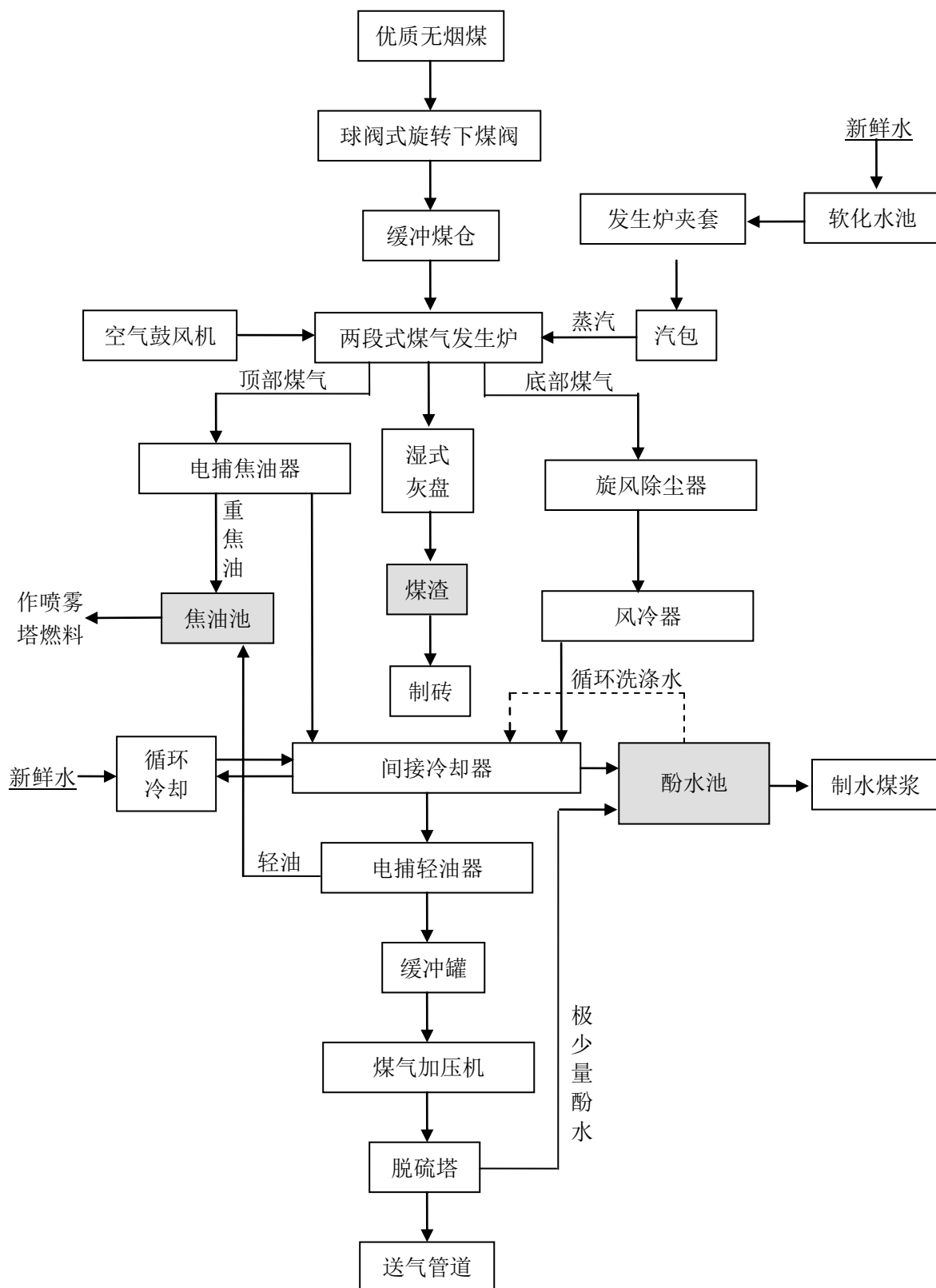
图 2.2-5 煤制气工艺流程图
