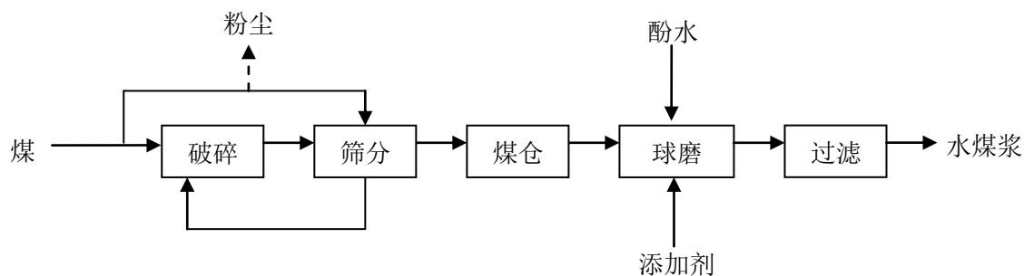
图 2.2-6 水煤浆生产流程图
