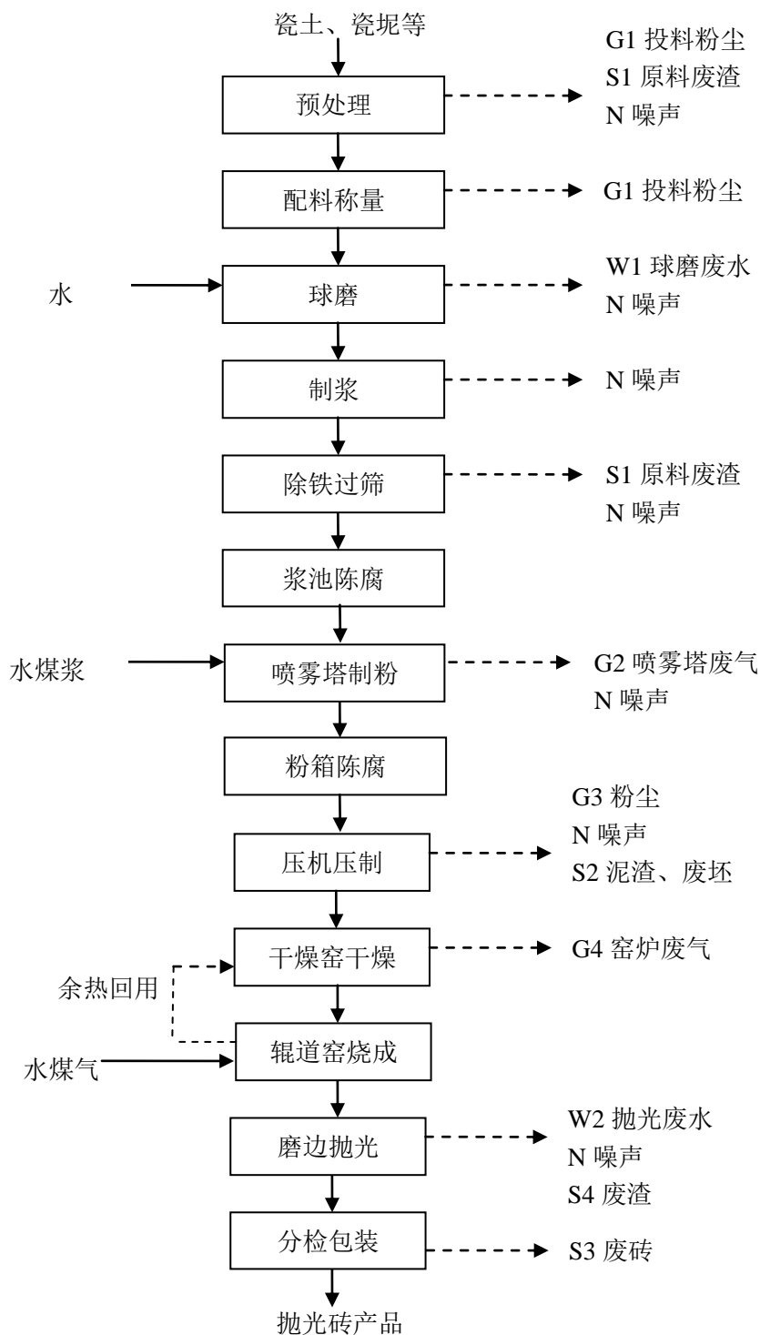
图 2.2-1 粉料制作工艺流程图
