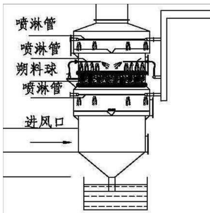
图 2.2-12 湍球脱硫塔结构图
