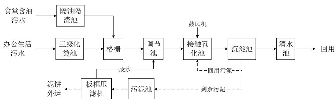
图 2.2-9 项目生活污水处理工艺流程图
