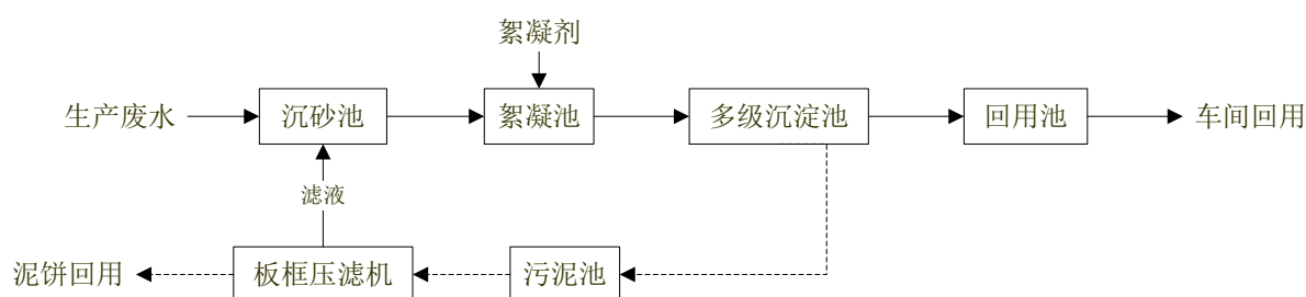
图 2.2-7 生产废水混凝沉淀处理工艺流程图
