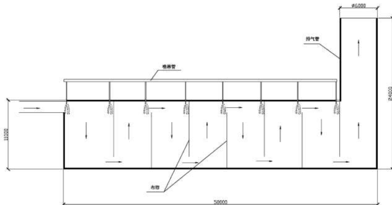
图 2.2-11 碱液喷淋室结构图
