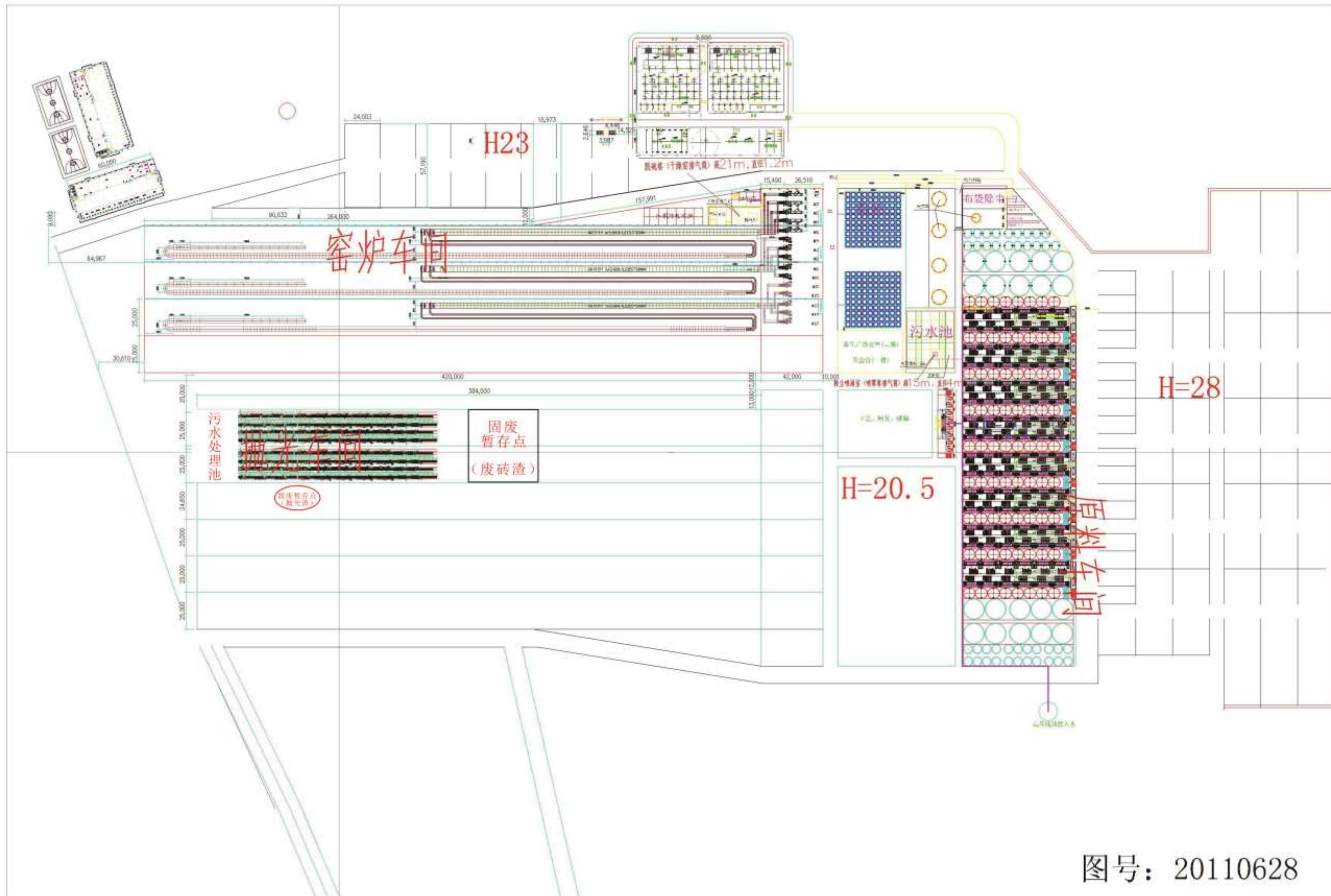
附图 4：厂区平面布置图：
