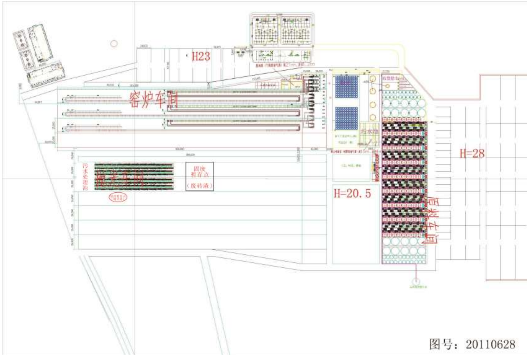
图 2.1-3 本项目平面布置图
