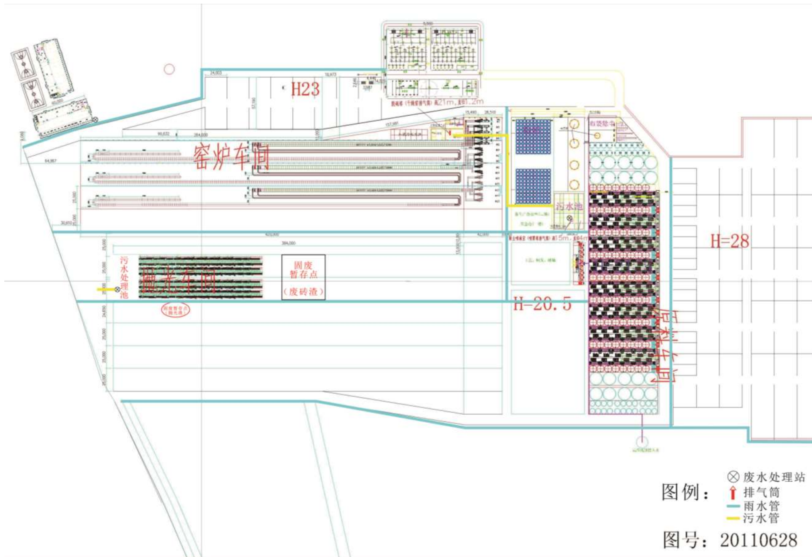
附图 5: 雨、污水流向图:
