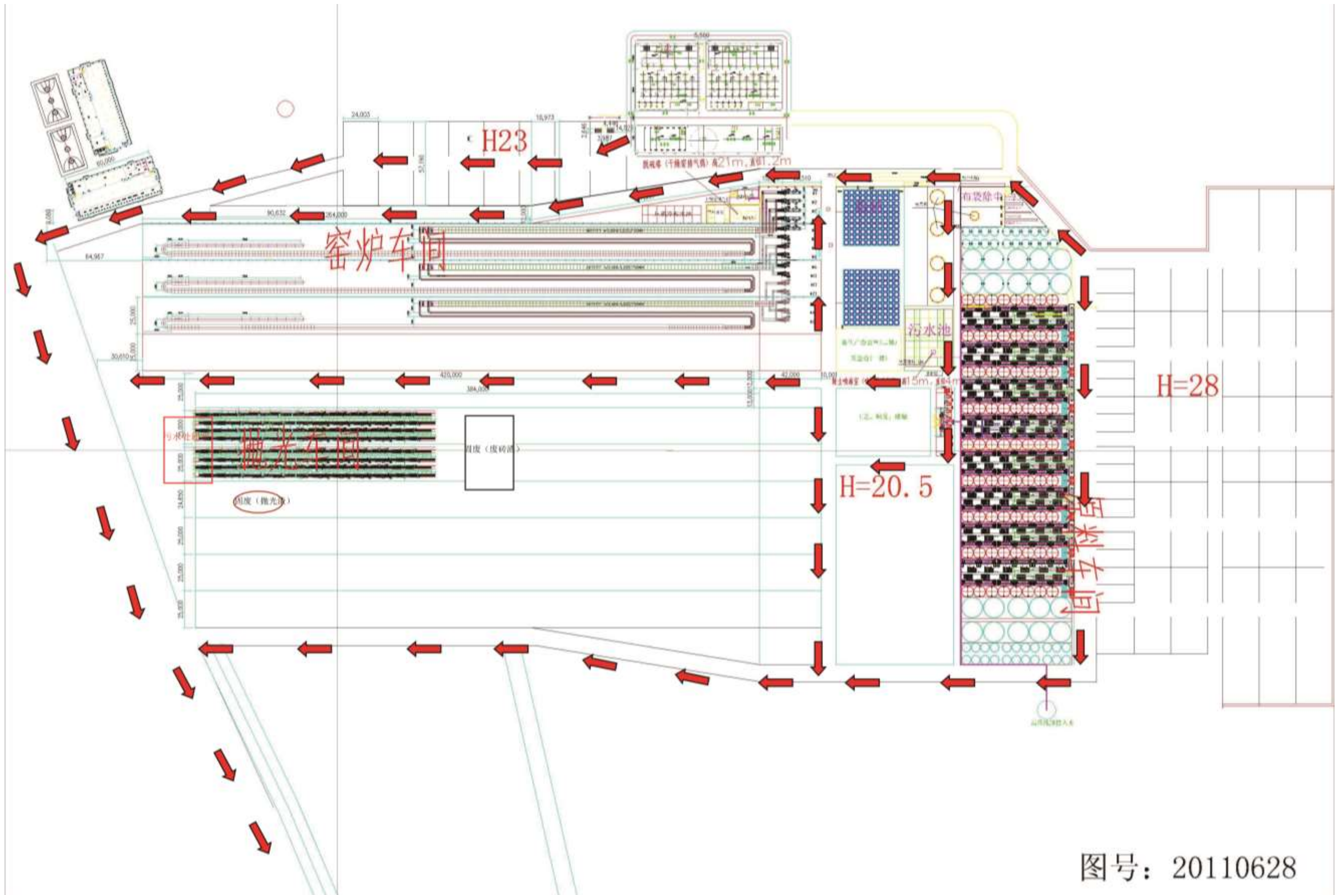
附图 6: 紧急疏散路线图:
